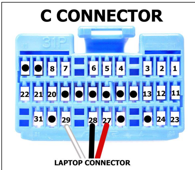
Connector PN 430020
